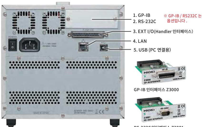
본체 뒷면 (인터페이스는 5 모델 공통)
