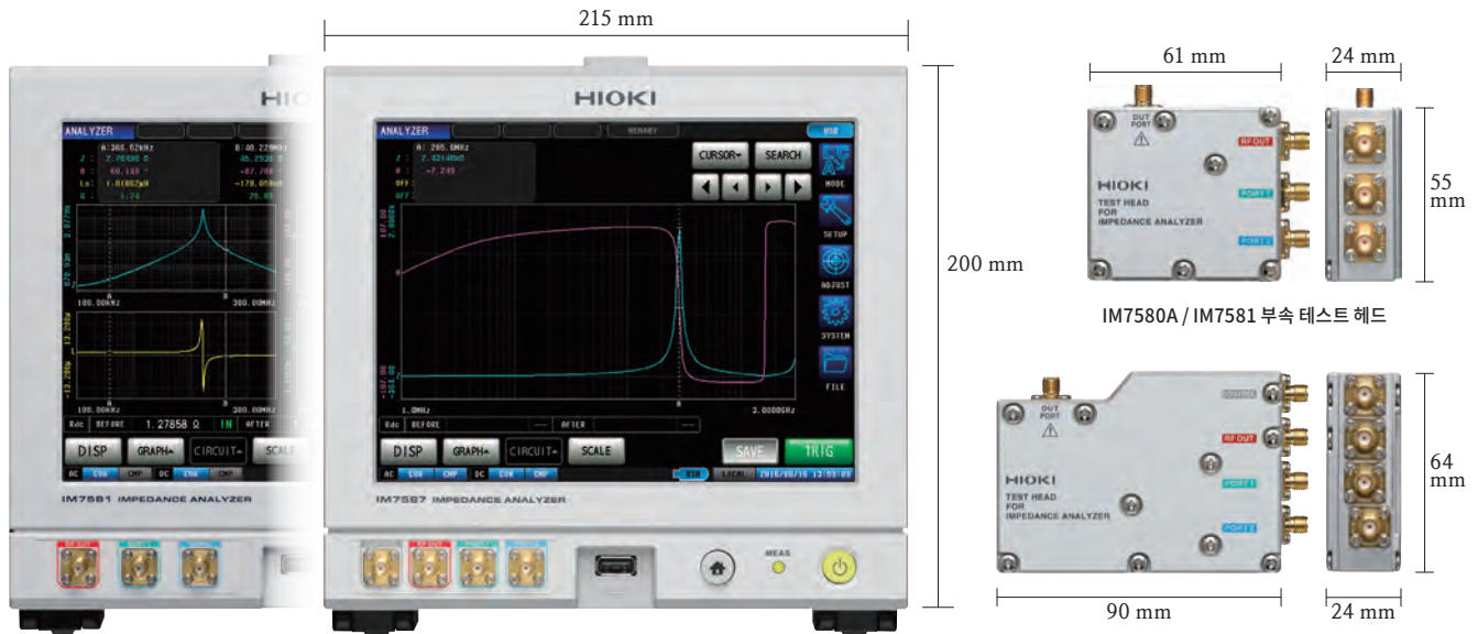
IM7581 본체 정면 (※ IM7580A 와 공통)
